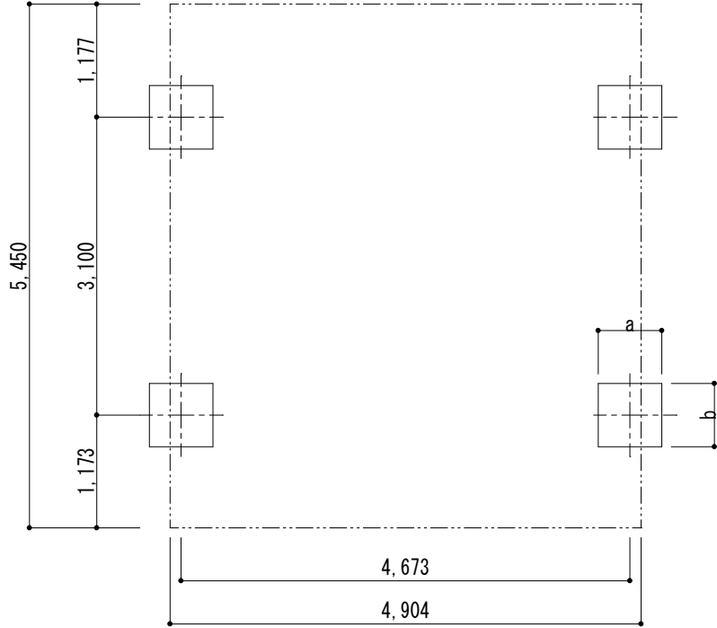
■ 基礎配置図
